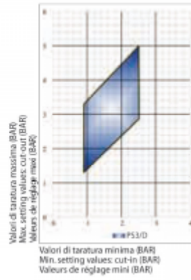
Grafico di taratura PS/3
