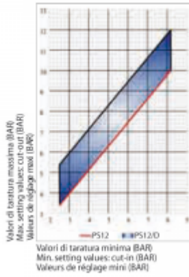
Grafico di taratura PS/12 + PS/12D
