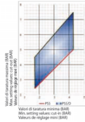
Grafico di taratura PS/5 + PS/5D
